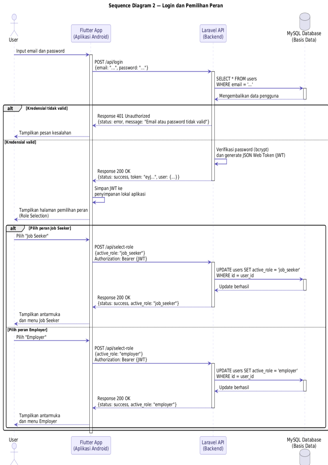
gambar 9.sequence login dan pemeilihan peran
