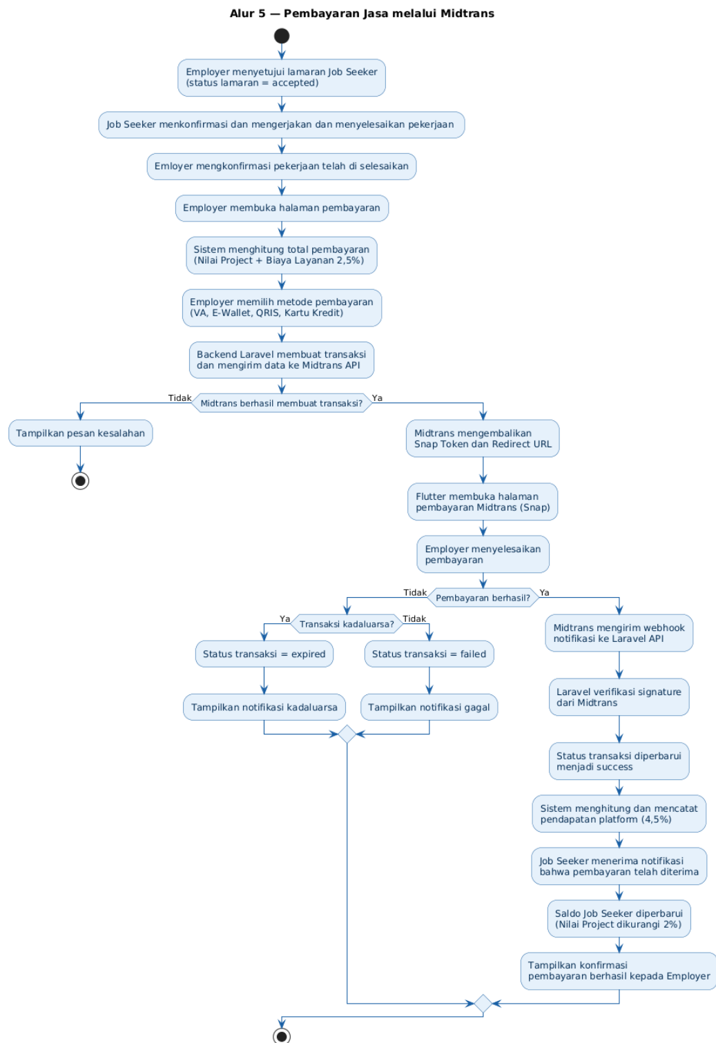
gambar 7. Activity diagram pemebayaran jasa
