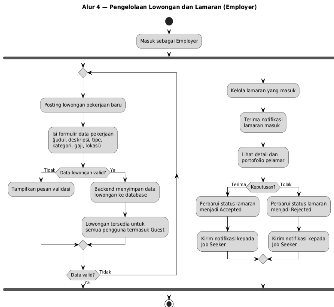
gambar 6. Activity diagram pengelolaan lowongan pekerjaan
