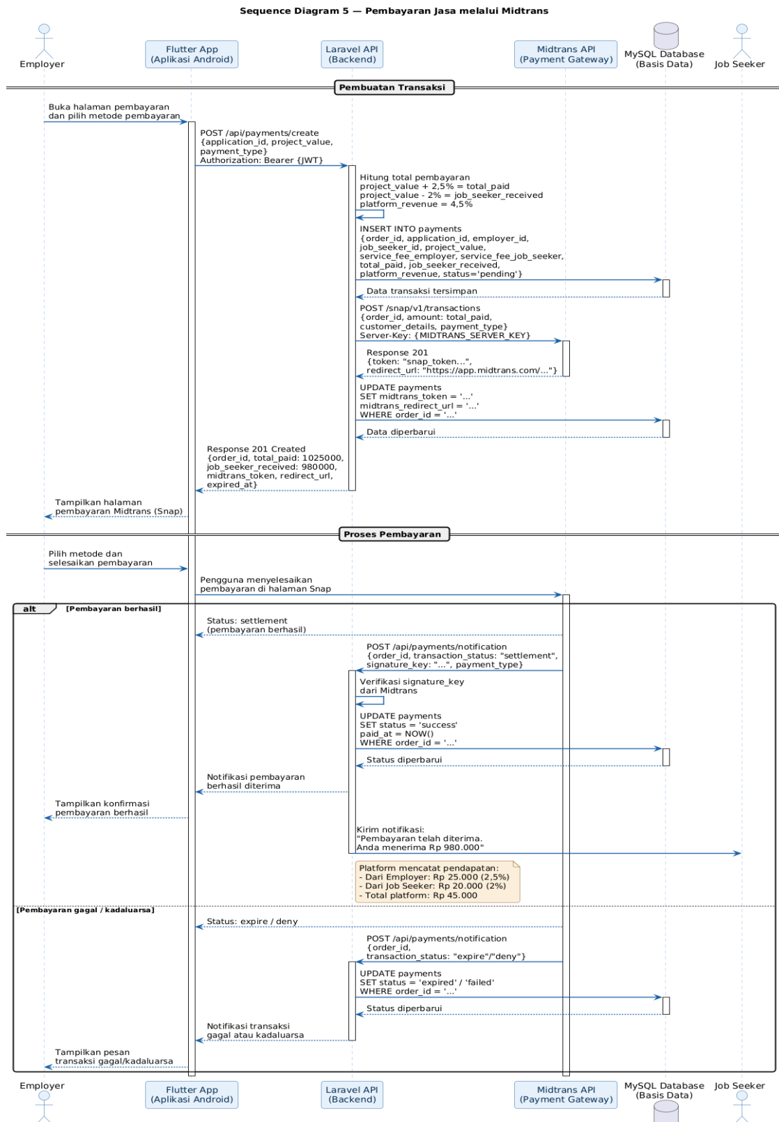
gambar 12.sequence diagram pembayaran jasa
