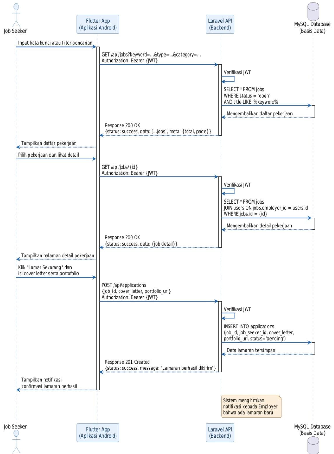
Sequence Diagram 3 — Pencarian dan Lamaran Pekerjaan (Job Seeker)
